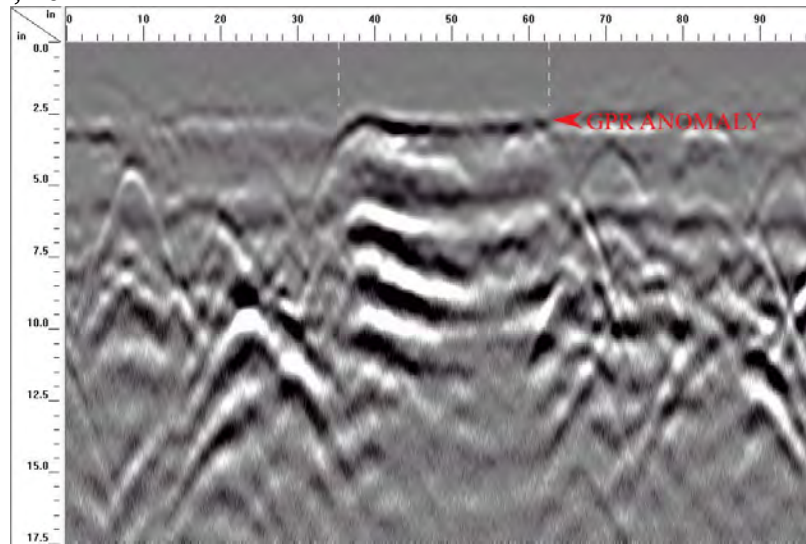
GPR Data 2
