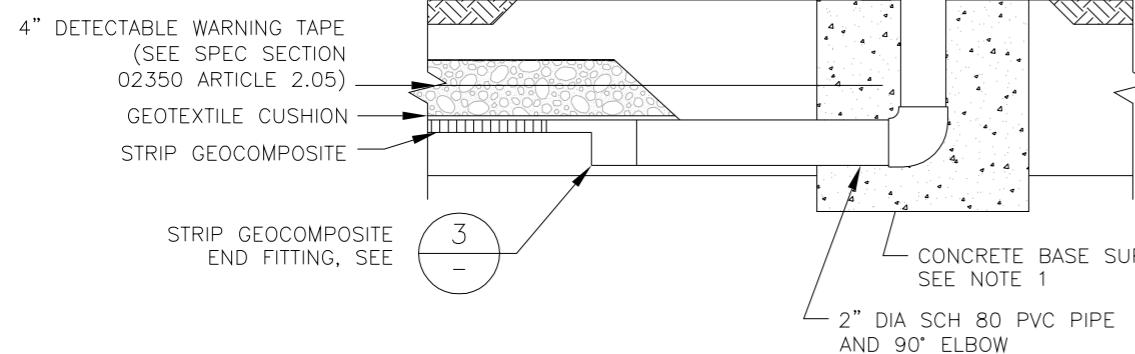
2 LFG VENT RISER DETAIL SCALE: NTS
