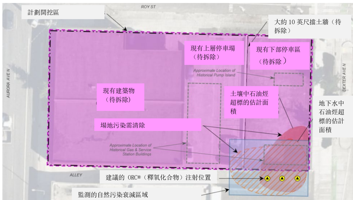
圖 3. 顯示歷史和現有結構位置、污染區域和計劃挖掘區域的清理工作站點地圖。
